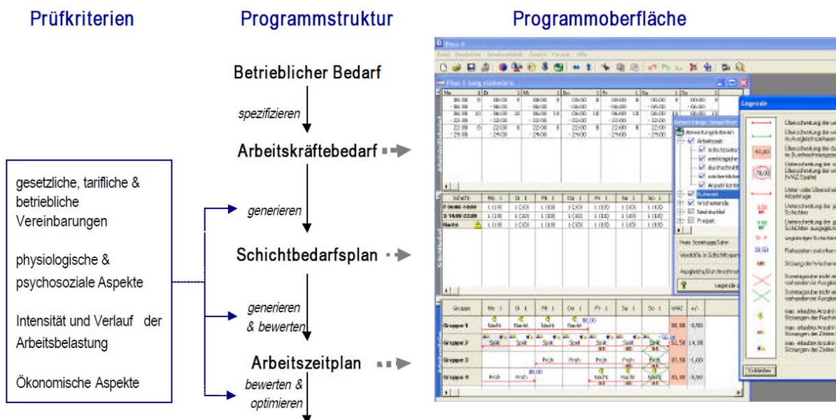
Abbildung: Programmstruktur und Programmoberfläche von BASS 5
